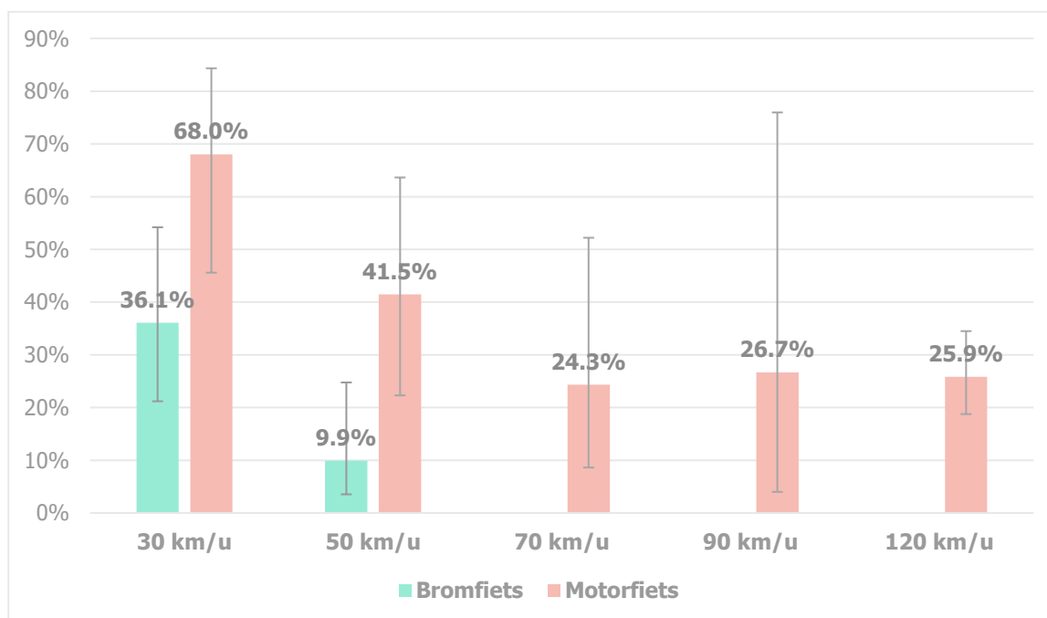
Grafiek 16 Gewogen percentages met schatting van de betrouwbaarheidsintervallen (CI 95%) van de chauffeurs in snelheidsovertreding volgens het snelheidsregime en het type G2W.
