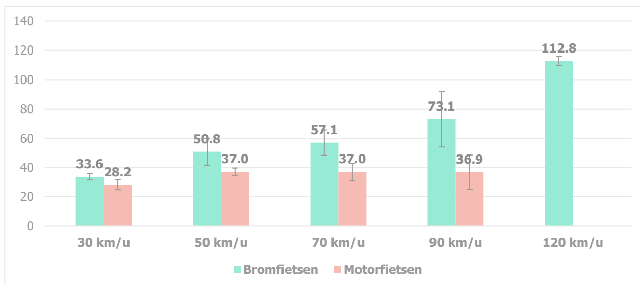
Grafiek 15 Gewogen gemiddelde snelheid met betrouwbaarheidsinterval, volgens het type G2W en per snelheidsregime. Voor bromfietsers geldt een wettelijke limiet van 25 of 45 km/u, voor motorfietsen niet.
